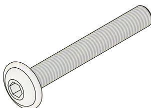
22 X L HEX BOLT M6 H4 Ø6 L45mm 636 M8 075
