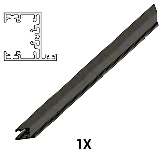
1X HORIZONTAL DOOR PROFILE 733 HOR 1000 501
