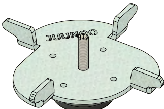
14X JUUNOO LEVELPLATE + FOOT 710 A 150XM10 + FOOT
